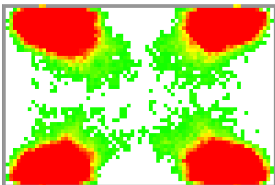
Abbildung 48: Dichteplot Schritt 1
