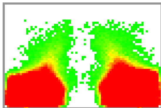
Abbildung 49: Dichteplot Schritt 2
